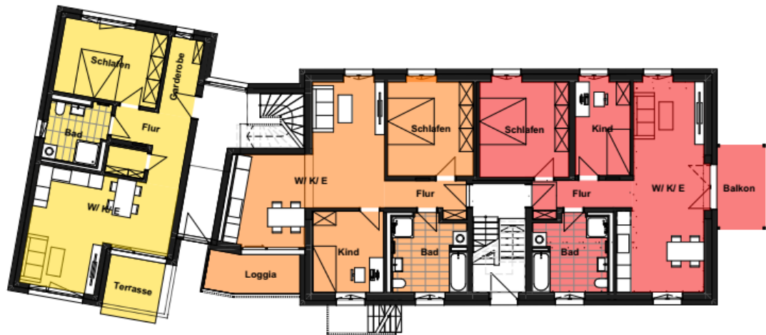
Neubau EG Wohnung 3 ca. 64m 2
